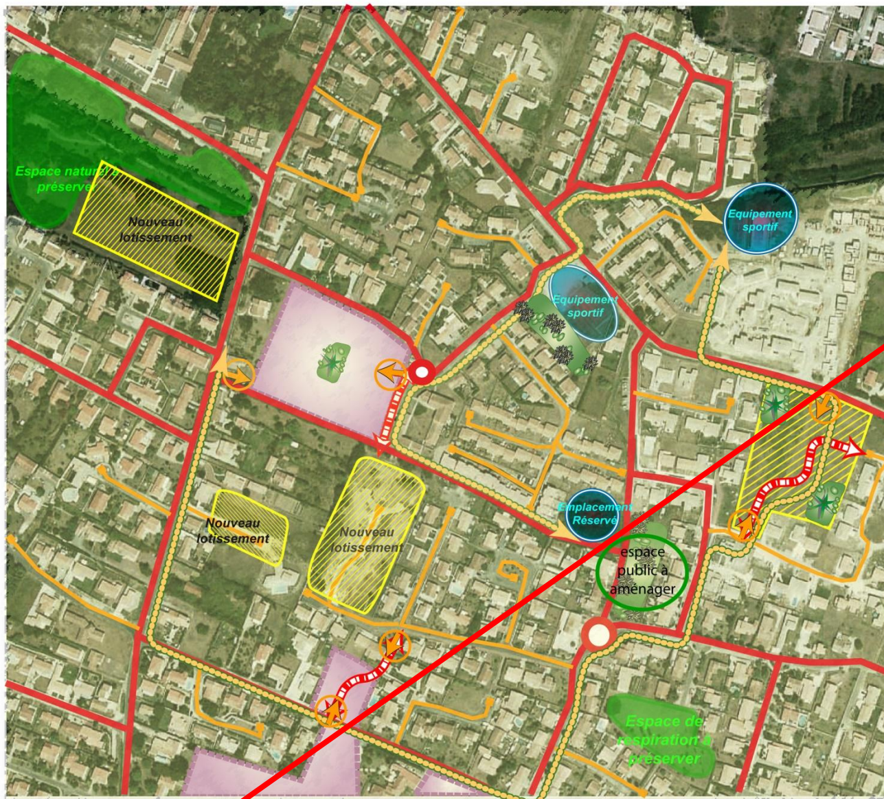
Profils de voirie à créer ou réaménager (exemple non exhaustif)
